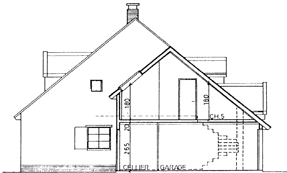
COUPE BB
