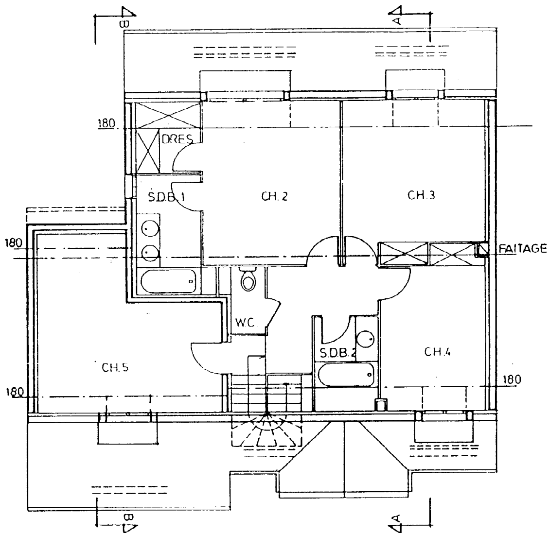
PLAN ETAGE
