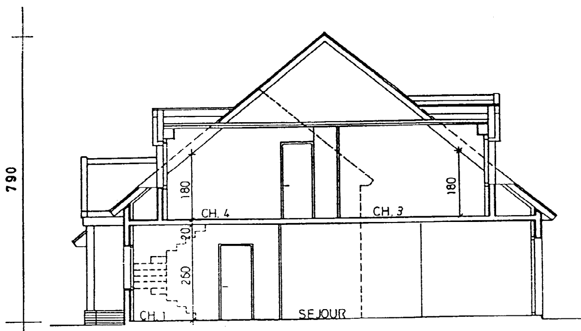
COUPE AA
