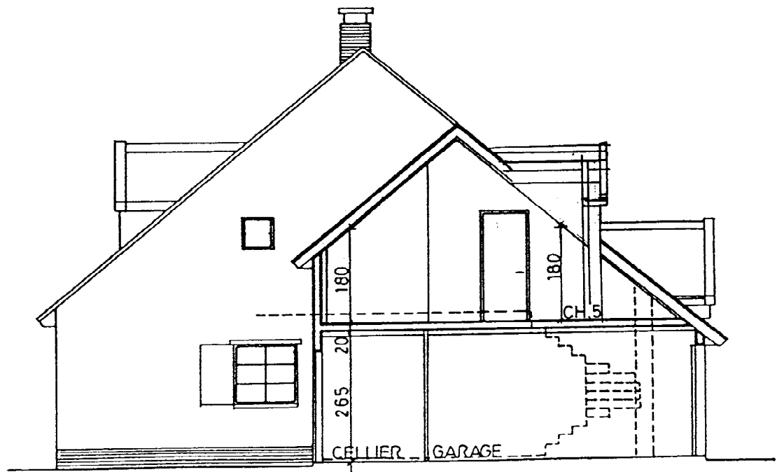
COUPE BB
